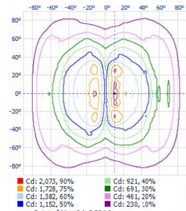
Isofootcandle Plot
